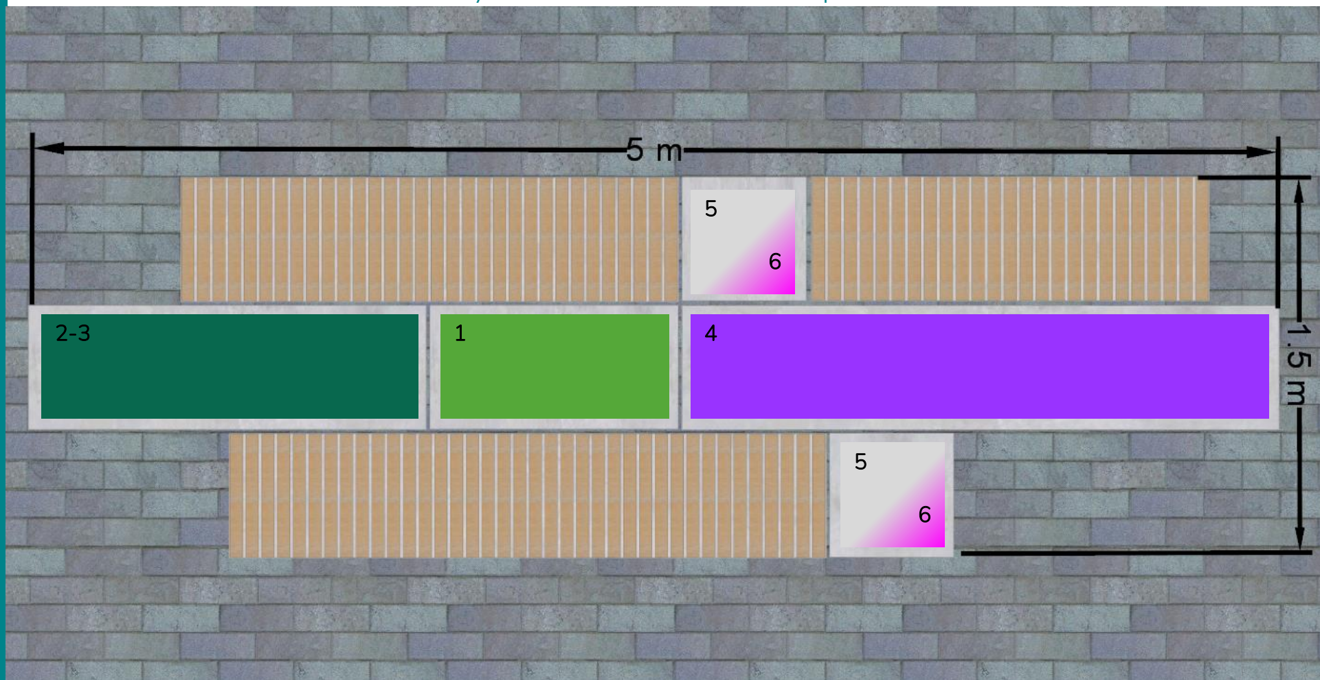
Схема установки МАФ и посадки растений
